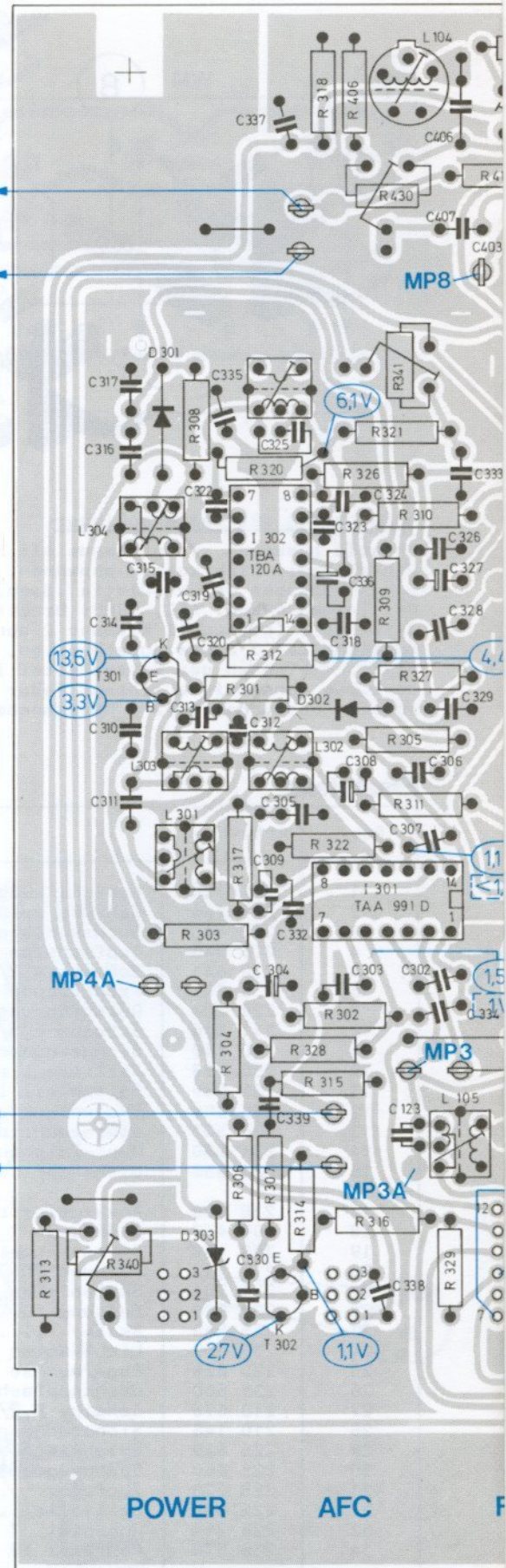
Fig. 3 HF-Platte
