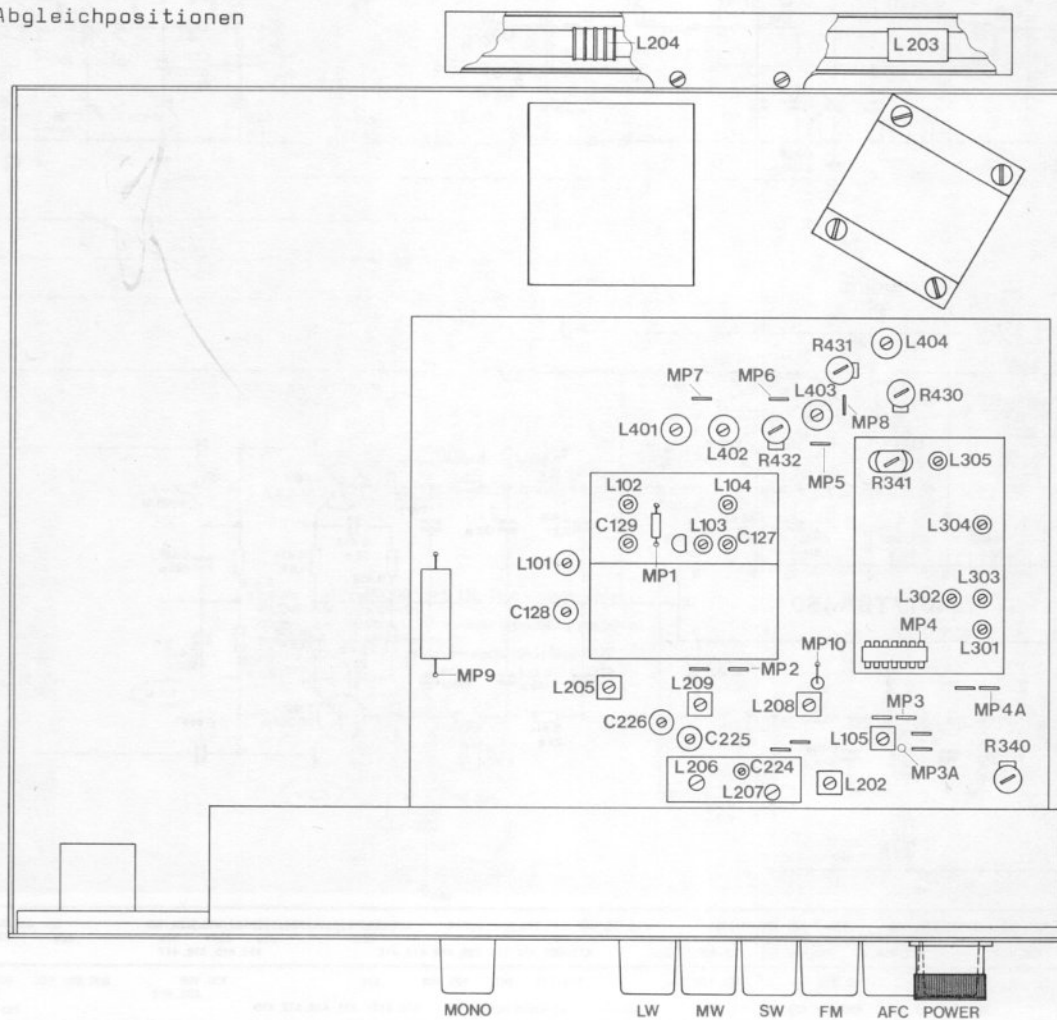
Fig. 1 Abgleichpositionen
